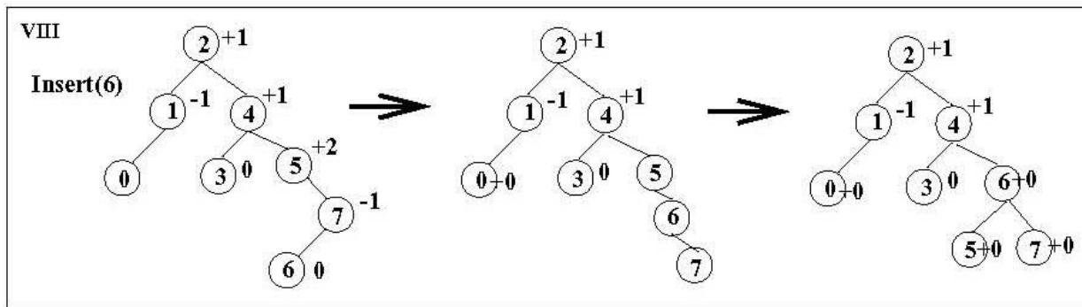
Vložení prvků {1,2,3,4,5,0,7,6} do AVL stromu
