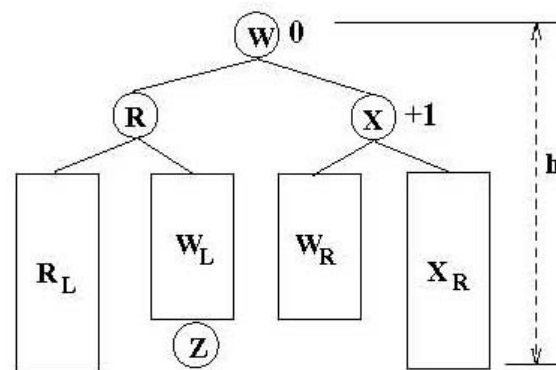
Strom po levé rotaci v R
