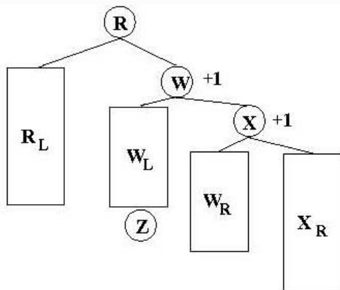
Strom po pravé rotaci v X
